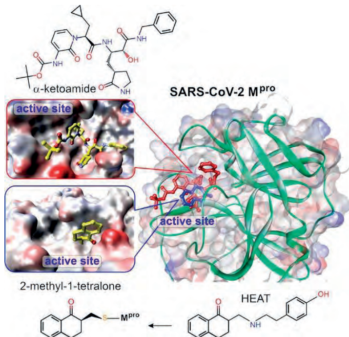
Abb.1: Röntgenstruktur der SARS-CoV-2-Hauptprotease M pro mit an das aktive Zentrum gebundenem α-Ketoamid- (rot) [2] oder 2-Methyl-1-Tetralon-Inhibitor (blau) [3]. Auf der linken Seite sind die Topologie und die elektrostatische Ladungsverteilung der Bindungsstellen dargestellt. Die 2-Methyl-1-Tetralon-Gruppe ist durch chemische Reaktionen von M pro und HEAT an das aktive Zentrum gebunden [3].
