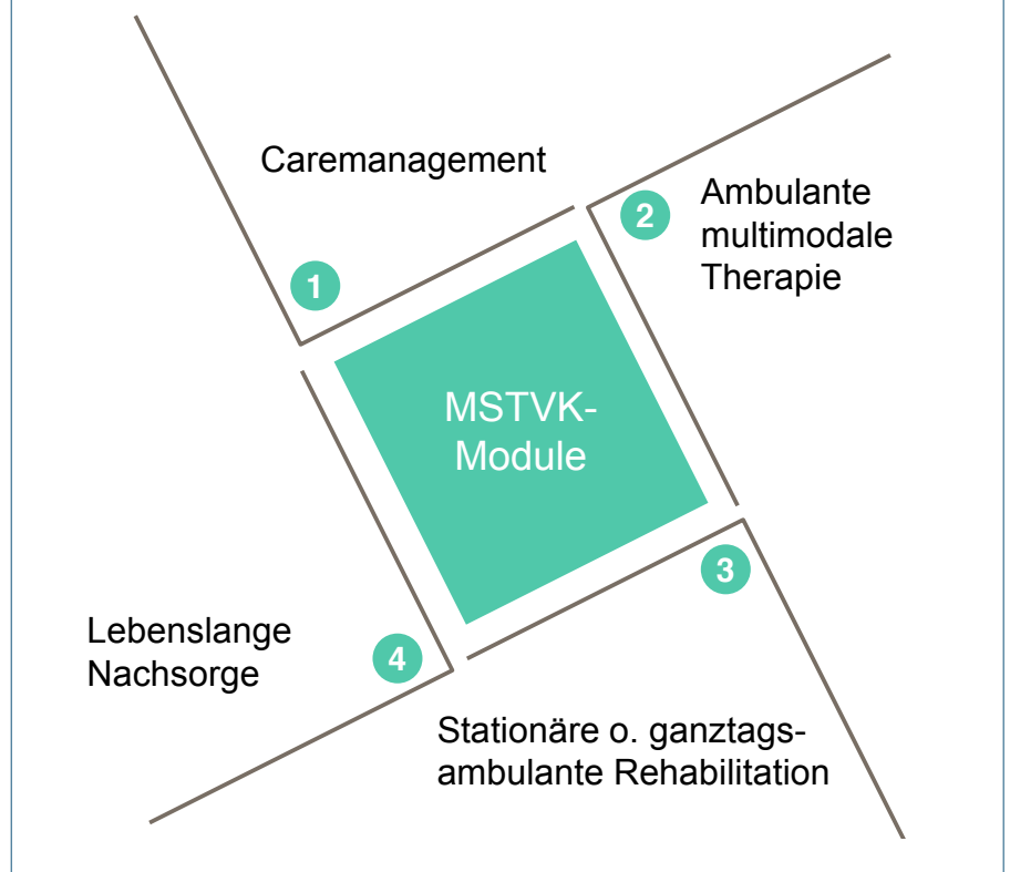
ABBILDUNG 1: Projektmodule
